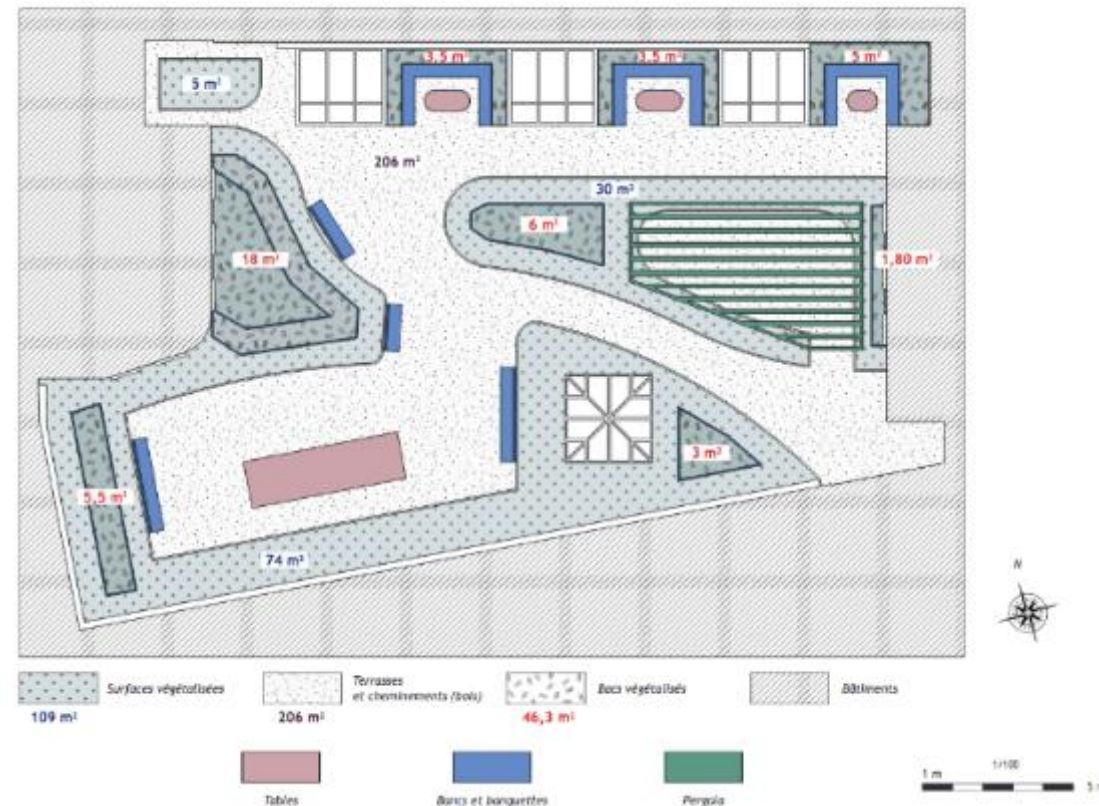
Plan masse – Surfaces et plan des sols
